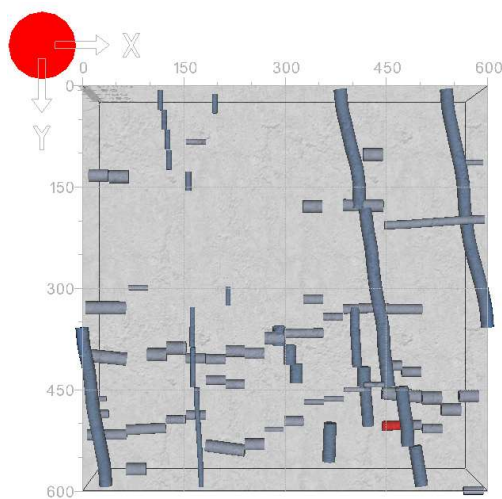
Πλάκα 1 (κάτοψη).
