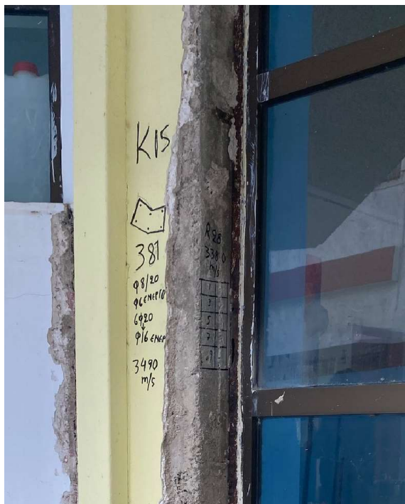
Υποστύλωμα K15
