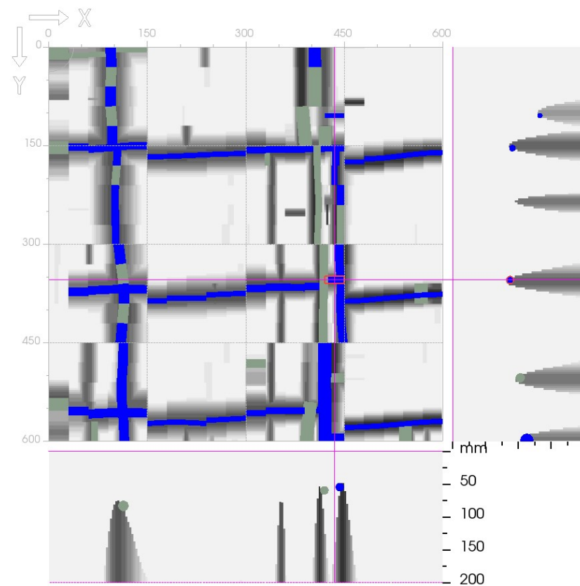
Υποστύλωμα K5.
