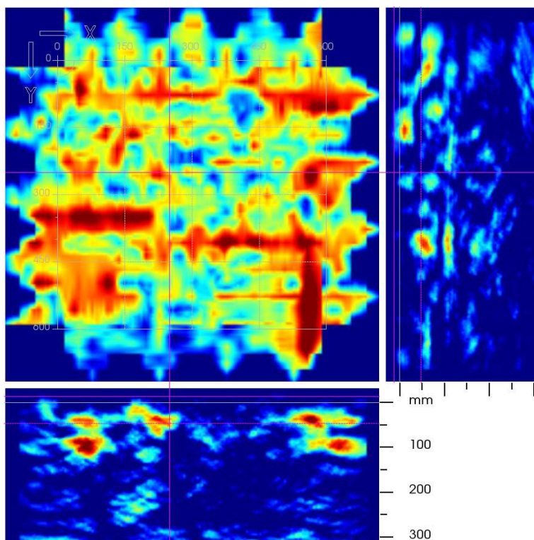
Υποστύλωμα Κ5.
