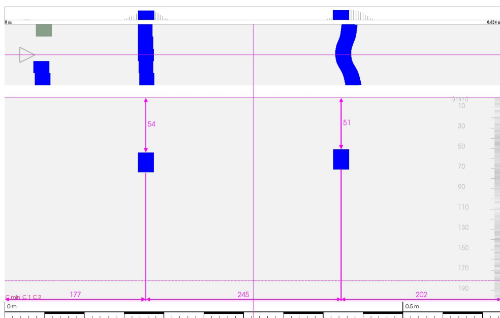
Υποστύλωμα K22.
